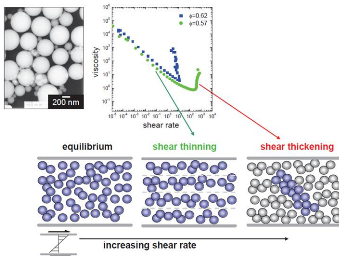
Kuva 1. STF-nesteen toimintaperiaate.
