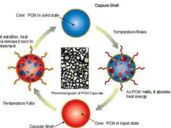
Kuva 2. Faasimuutosmateriaalin toimintaperiaate.
